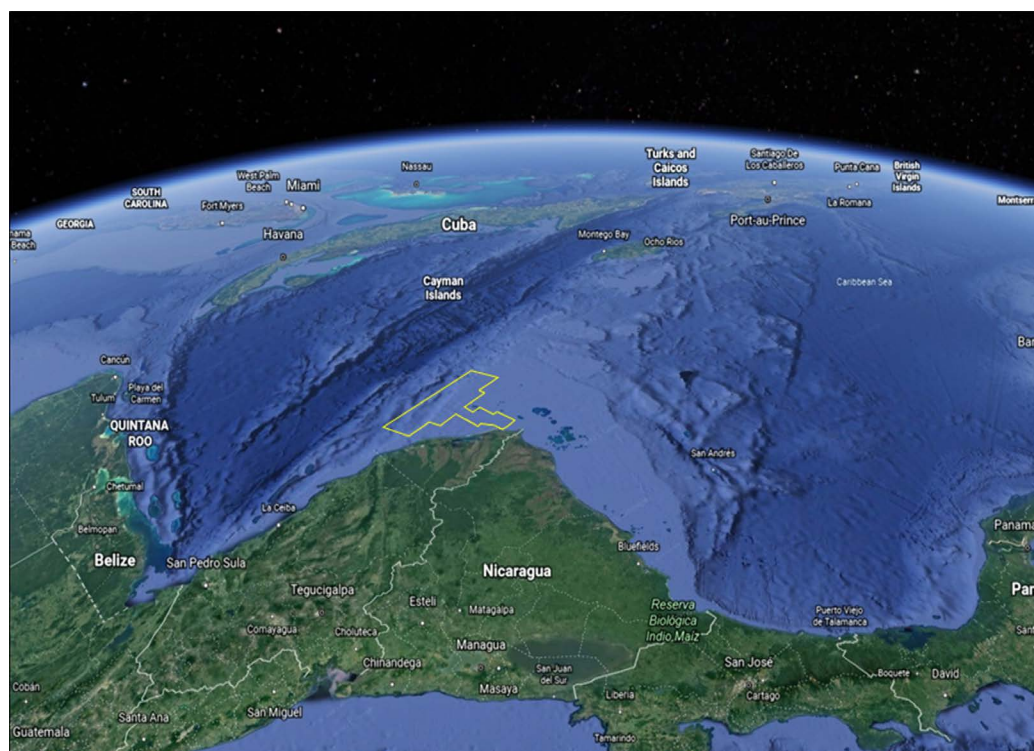
El sitio de mayor referencia es el pozo Main Cape, en la cuenca de La Mosquitia, que ha dado muestras claras de petróleo de 38 grados API (por sus siglas en inglés American Petroleum Institute).
